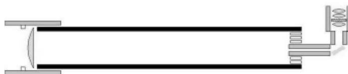
Figura 1 - Esquema da luneta proposta, mostrando, na extremidade direita, o conjunto de lentes formando a lente ocular, e na extremidade esquerda a lente objetiva.
